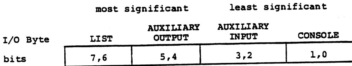
Figure 4-3. I/O Byte
