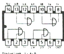
Positive Logik T. A. B
